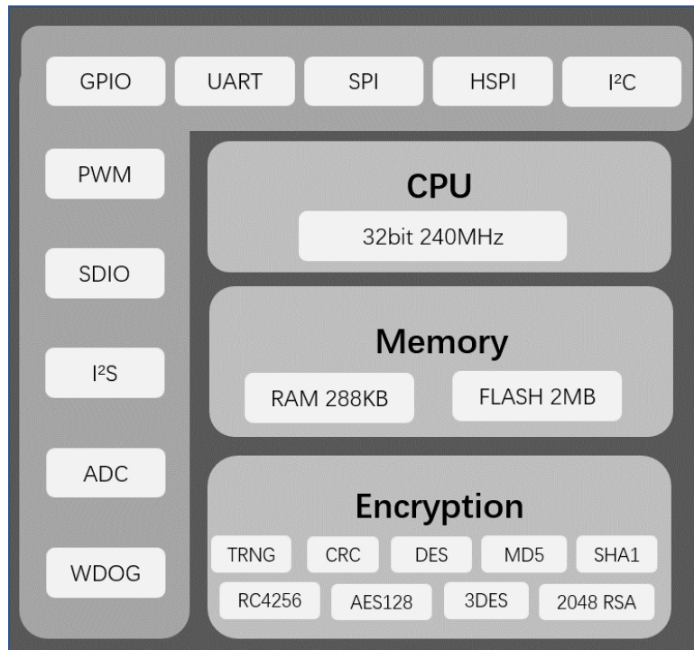
图 3-1 W805 芯片框图
